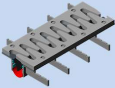
이물질방지 이중배수핑거조인트 (특허 제 10-2042954 호)
