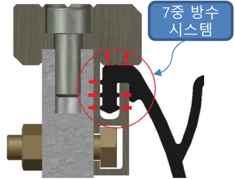
7중 방수 시스템
