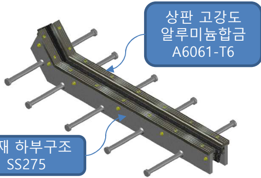
분리형 레일조인트
