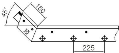
측면도
